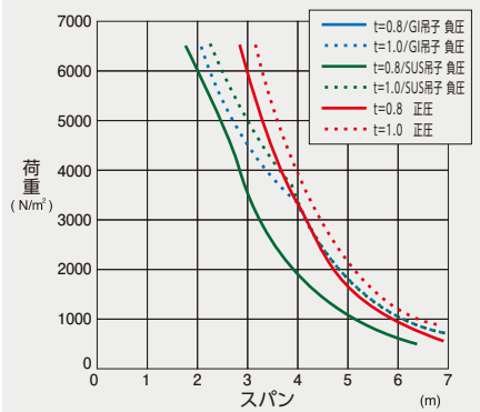
連続梁
